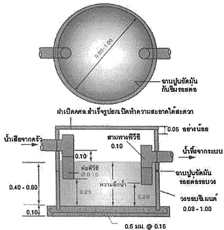
ภาพที่ : ๑ บ่อดักไขมันแบบวงอบซีเมนต์
